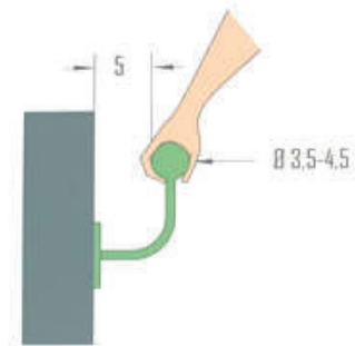
적합한 핸드레일의 설치
